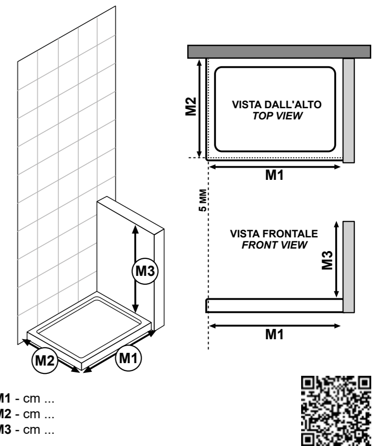
"M" - Spazio in angolo con muretto Dx Corner shower enclosure with low wall to the right. Eck-Duschkabine mit niedriger Mauer rechts. Cabine de douche en angle avec muret bas à droite.
