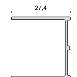
PROFILO A MURO WALL PROFILE - WANDPROFIL - PROFIL DE MUR
