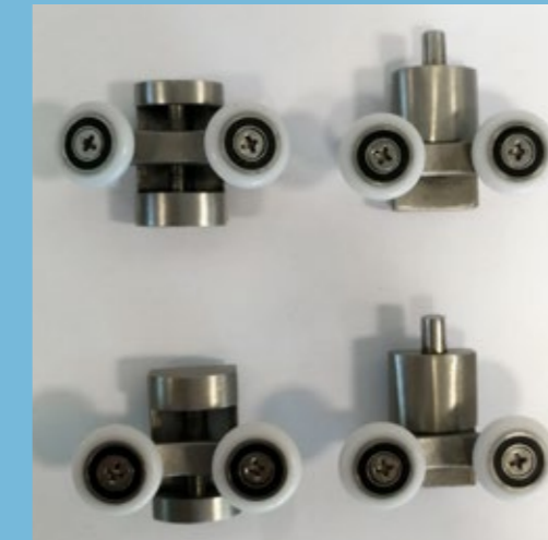
PANAREA / ORTIGIA CARRUCOLE - ROLLERS RIEMENSCHLEIBE - ROULETTE
