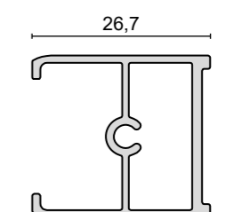
PROFILO A MURO WALL PROFILE - WANDPROFIL - PROFIL DE MUR
