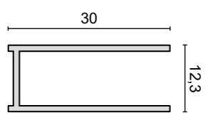
PROFILO A MURO WALL PROFILE - WANDPROFIL - PROFIL DE MUR
